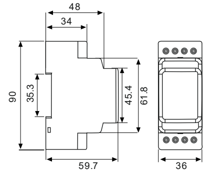
Size (Type PK 28)
